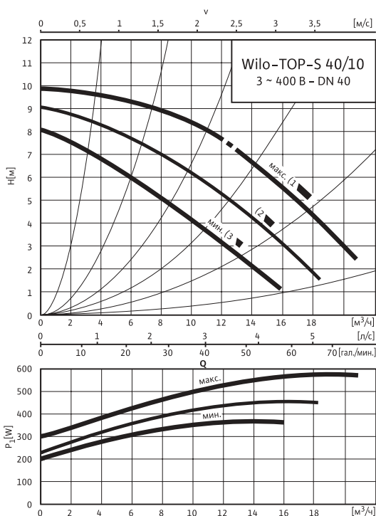
Характеристики Wilo-TOP-S
