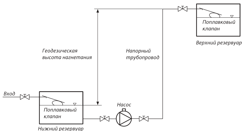
Насосная система для подачи воды на высоту
